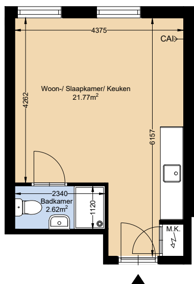
10e Verdieping
