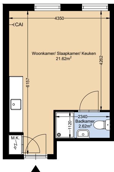
9e Verdieping
