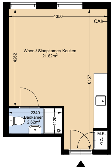
12e Verdieping
